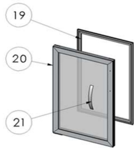
PUERTAS DE CRISTAL MODELO DEBP GLAZING DOOR MODEL DEBP
